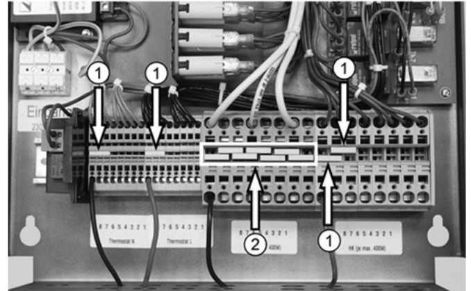
Abb. 8: Beispiel neu gesetzter Brücken bei einer benötigten Leistung von 3x400 VA = 1200 VA
