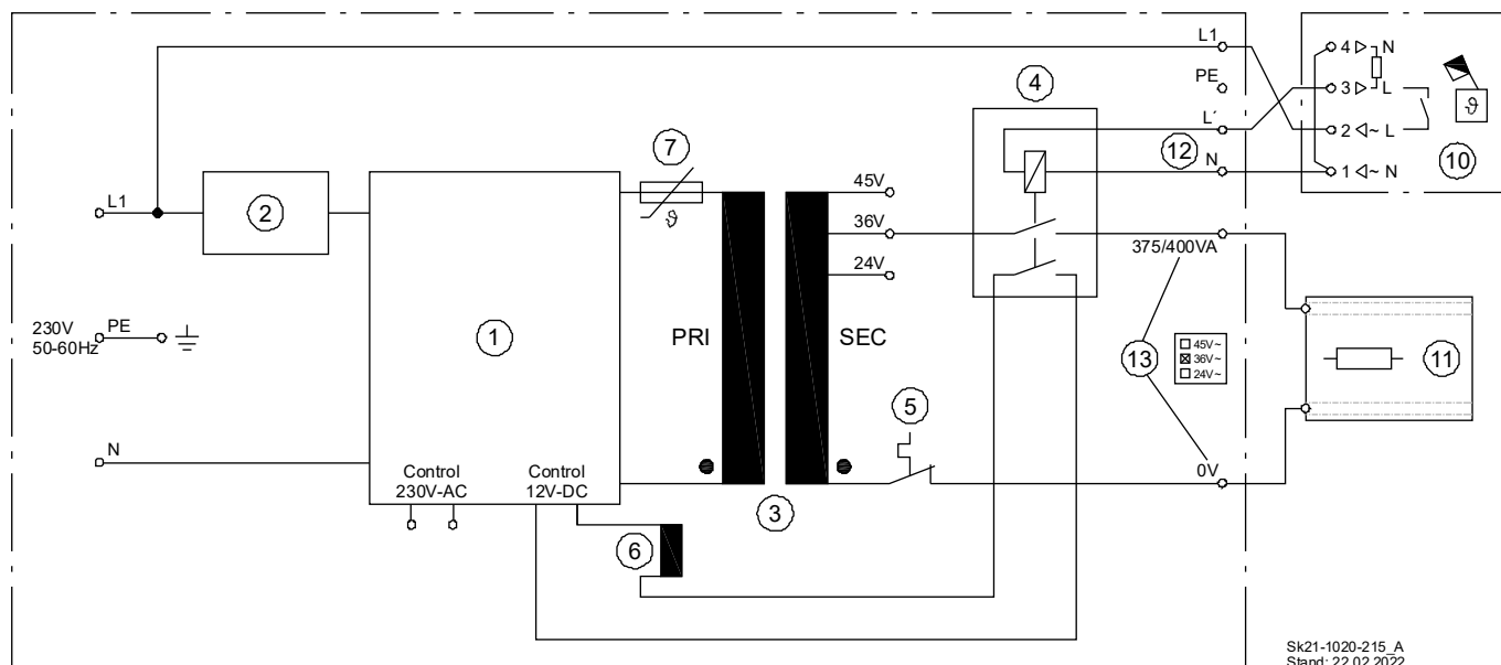
Abb. 12: Stromlaufplan – Ausführung für 800-1200 VA
